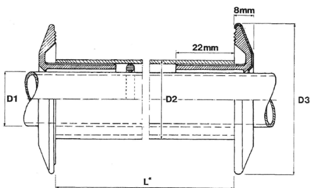
Rosétbøsningssæt VVS nr. 01 5500.6--/01 5503.6-- består af: 2 rosétbøsninger VVS nr. 01 5500/01 5503 1 bøsningrør VVS nr. 01 5546 1 neoprenpakning VVS nr. 01 5520
