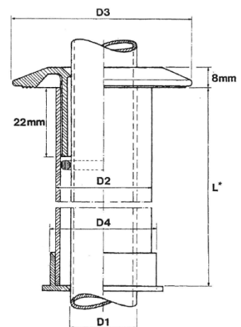
Rosétbøsningssæt VVS nr. 01 5500.8--/01 5503.8-- består af: 1 rosétbøsning VVS nr. 01 5500/01 5503 1 bøsningrør VVS nr. 01 5546 1 neoprenpakning VVS nr. 01 5520 1 pudsring VVS nr. 01 5551
